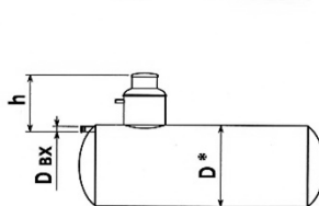
Горизонтальная установка
